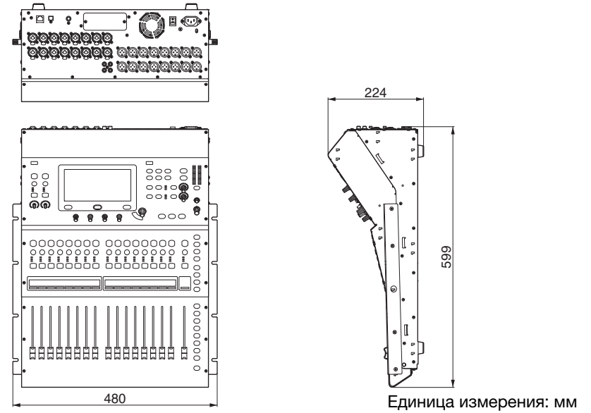
TF1 стоечного исполнения
