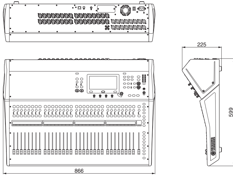
TF3
